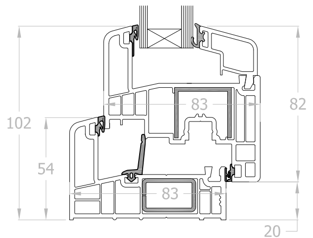
NODO INFERIORE FINESTRA E PORTAFINESTRA CON SOGLIA ALTA
