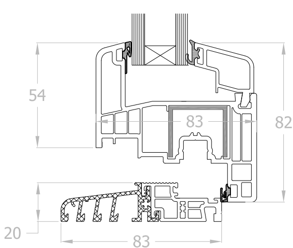
NODO INFERIORE PORTAFINESTRA CON SOGLIA RIBASSATA
